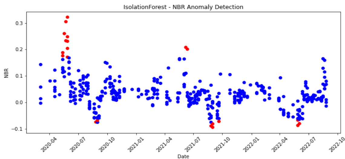
شکل ۸- نمودار تشخیص ناهنجاری NBR با روش جنگل جداساز
